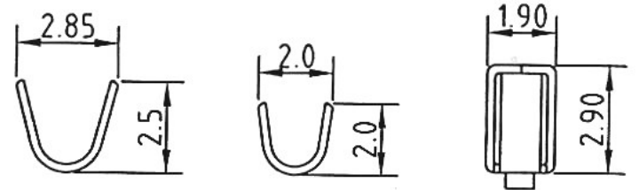
SECTION:A-A' SECTION:B-B' SECTION:C-C'
